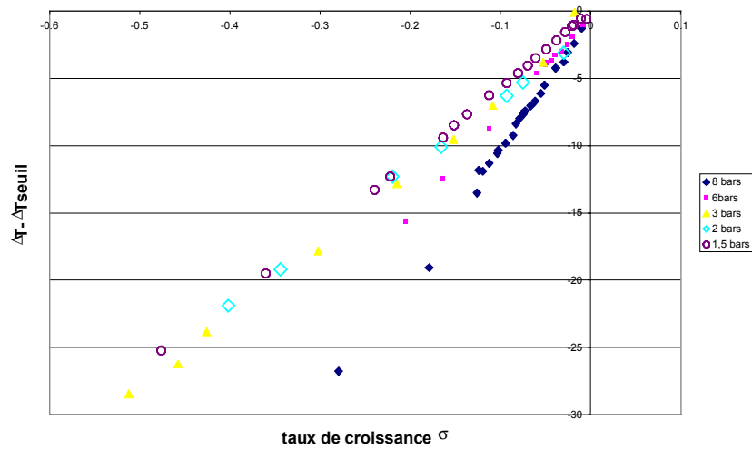
Fig 4: Evolution du taux de croissance en fonction de la pression moyenne.
