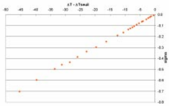
Fig 2 :Évolution de \sigma en fonction de l'écart au seuil pour P_{moyenne}=1,11 bars
