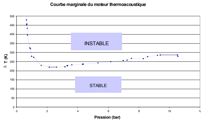
Fig 3 : Coupe de la surface marginale dans l'espace des paramètres ( P_{moyenne}, \Delta T )
