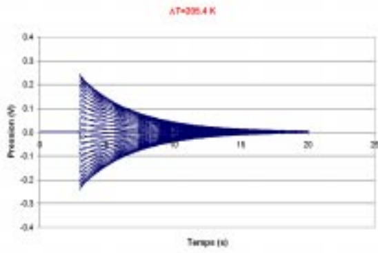
Fig 1 Réponse du moteur thermoacoustique à une sollicitation extérieure
