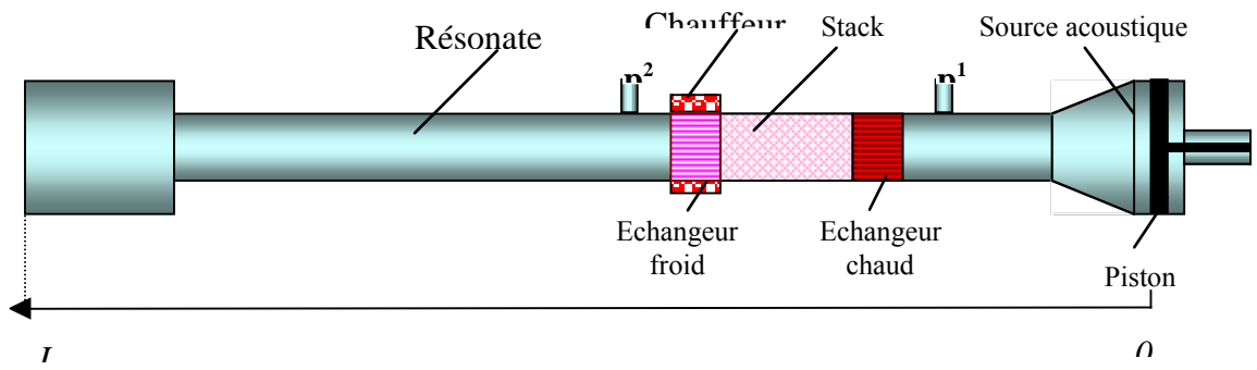
Figure 1 Réfrigérateur thermoacoustique avec gaz
