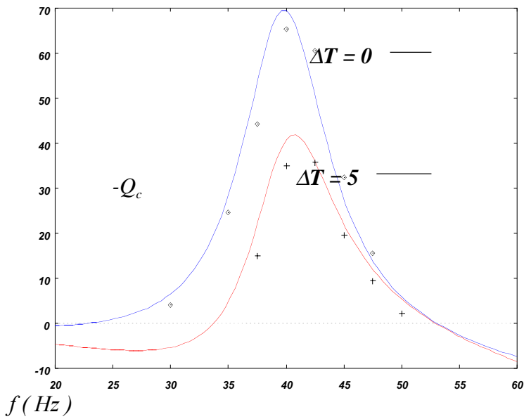
Figure 2: Puissance thermique pompée en fonction de la fréquence
