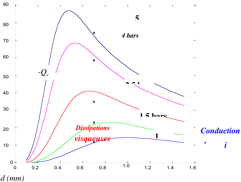
Figure 3 : Puissance thermique pompée en fonction de l'espacement entre plaques
