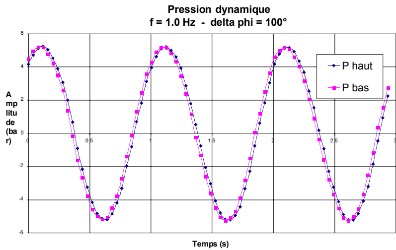
Figure 3 : Ondes de pression dans les deux chambres du réfrigérateur pour un déphasage de 100° entre les pistons et une pression moyenne de 20 bars.
