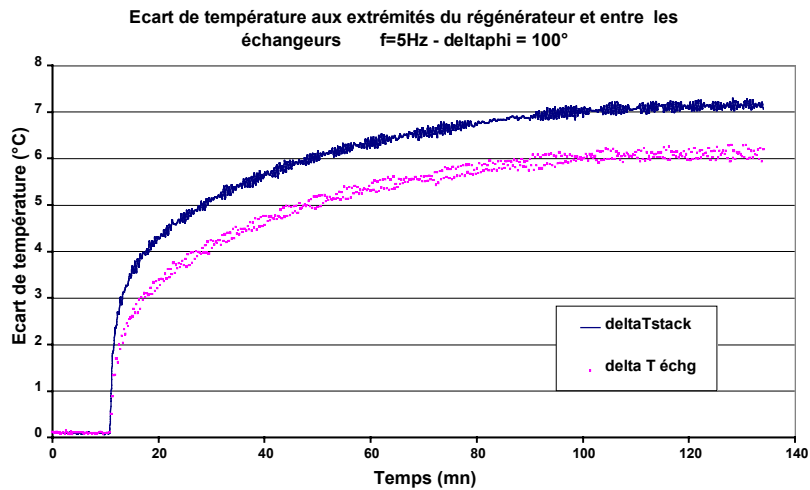
Figure 4 : Exemple de réfrigération.
